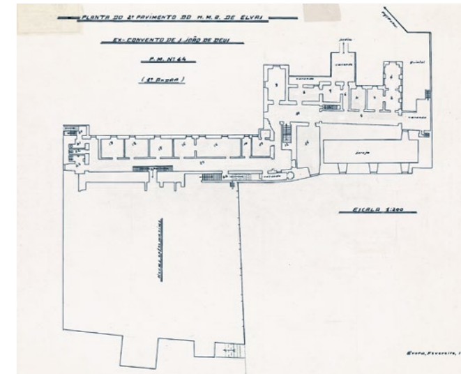
Sobrado, planta do Real Hospital Militar de S. João de Deus, Elvas, Portugal. Século XVIII. Upper floor plan, São João de Deus Royal Military Hospital, Elvas, Portugal. 18 th century.
