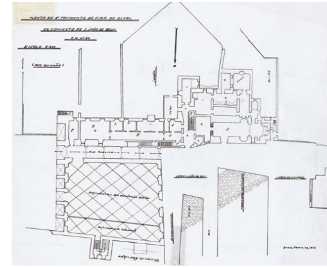
Piso térreo, planta do Real Hospital Militar de S. João de Deus, Elvas, Portugal. Século XVIII. Ground Floor plan, São João de Deus Royal Military Hospital, Elvas, Portugal. 18 th century.
